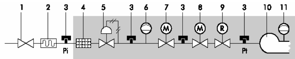
ОСНОВНАЯ ЛИНИЯ ПОДАЧИ ГАЗА
